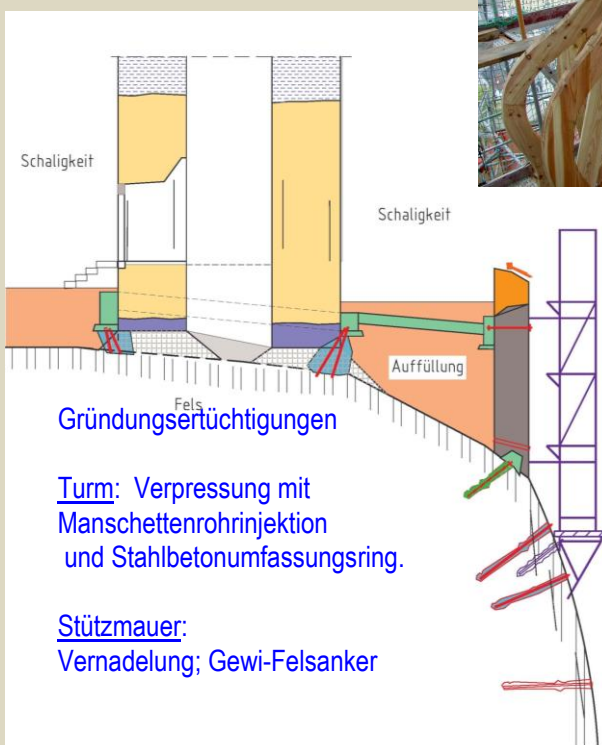
Ertüchtigung der Turmgründung
